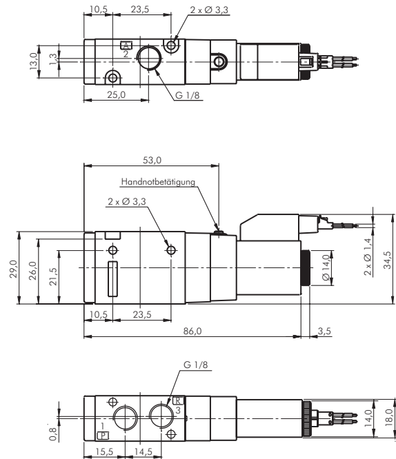
Typ mit 2-Pol-Stecker
