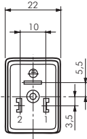
Maßzeichnung Typ CO 22-24V= DINB
