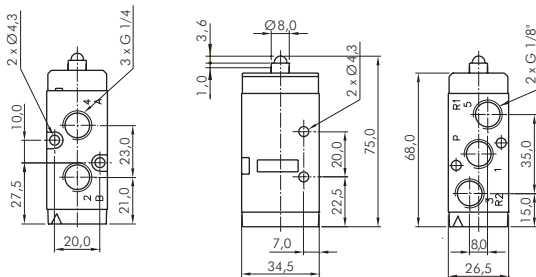
Typ PME410 MS
