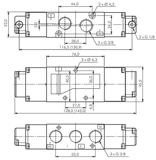
Typ SFP5200 (SFP5303, SFP5403, SFP5503)
