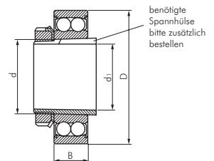
Typ 2RS Abgedichtet mit berührenden Dichtungen
