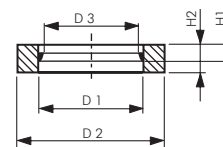
Typ O-Ring
