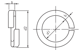
Form B (glatt)
