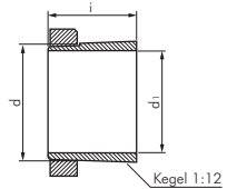
Spannhülse inkl. Mutter (Bitte separat bestellen)
