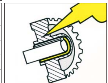
Typ 2RS Abgedichtet mit berührenden Dichtungen
