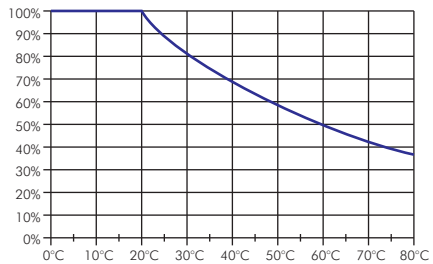
Druck/Temperaturdiagramm PUN-Schläuche
